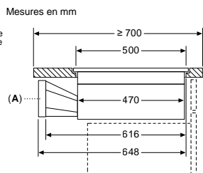
A: Adaptateur rond-plat
