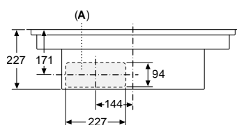
Mesures en mm Vue avant
