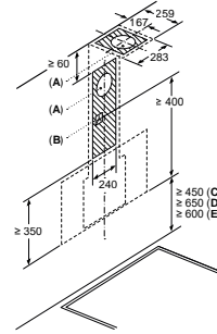
Mesures en mm
