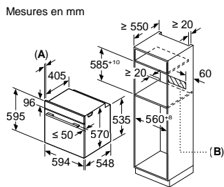
A: 19.5 mm B: Espace pour le raccordement de l'appareil 320 x 115 mm
