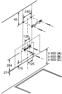
Mesures en mm Installation murale avec cheminée
