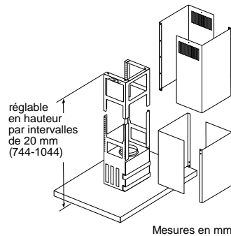
Mesures en mm
