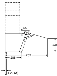
Mesures en mm
