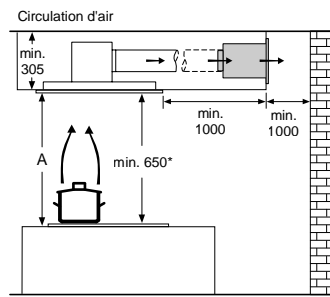
A : Performance optimale 700-1300 * À partir du bord supérieur du porte-casserole
