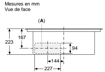
A: Connecté directement à l'arrière
