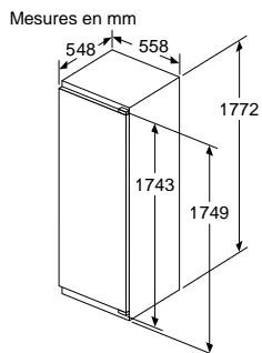
Mesures en mm
