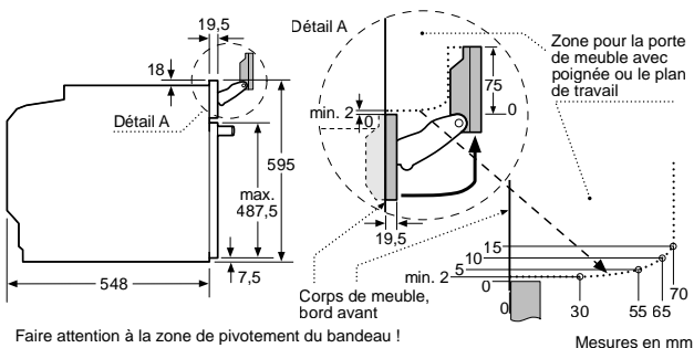
Mesures en mm
