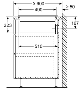
A: Connecté directement à l'arrière
