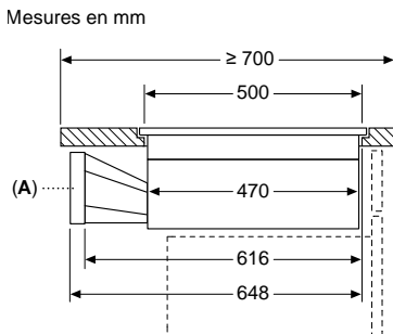
A: Adaptateur rond-plat
