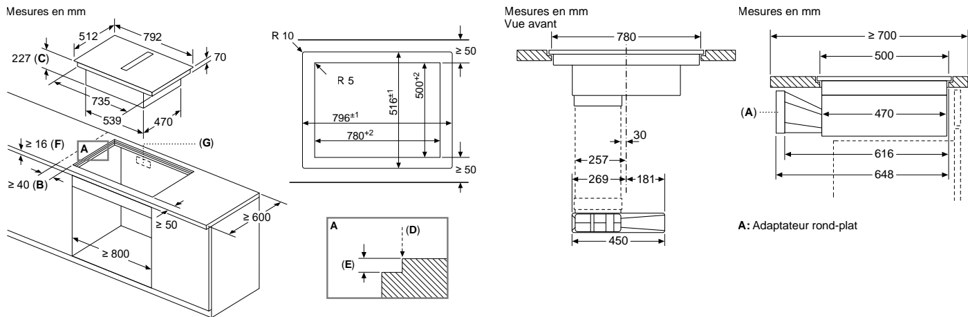
Mesures en mm Vue avant – découpage de l'unité pour la recirculation libre
