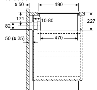
Mesures en mm Vue latérale
