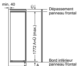
Mesures en mm
