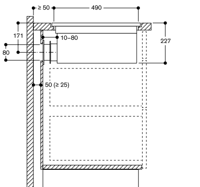
Vue de côté CV 282 101 en recyclage sans gaines - installation à fleur de plan
