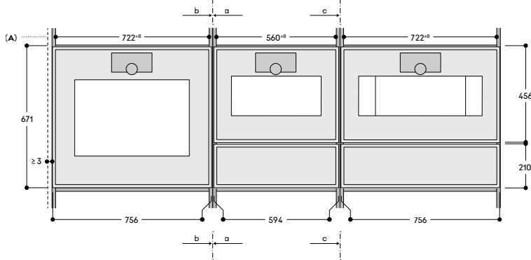
Vue latérale
