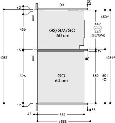
Vue latérale
