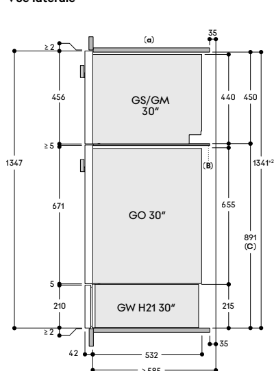
Vue latérale
