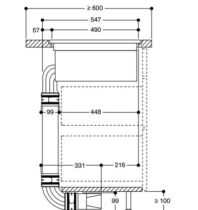
Vue de côté avec kit de recyclage pour un système avec gaines (coudes, gaines et diffuseur fournis) Profondeur plan de travail 600 mm - installation à fleur de plan
