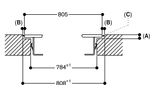
Coupe longitudinale
