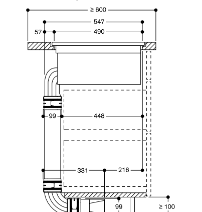
Vue de côté avec kit de recyclage pour un système avec gaines (coudes, gaines et diffuseur fournis) Profondeur plan de travail 600 mm (CA 082 061) - installation à fleur de plan
