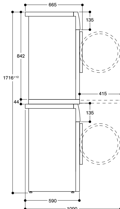
Vue latérale de WT 260 au-dessus de WM 260 avec kit d'installation
