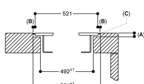
Coupe transversale
