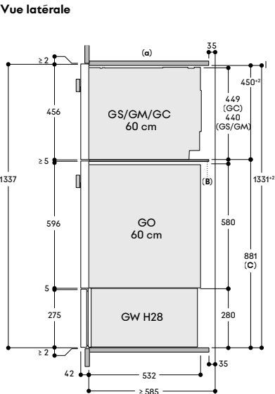
Vue latérale
