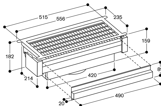
Tiroir extractible pour remplacement du filtre
