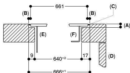
Coupe transversale
