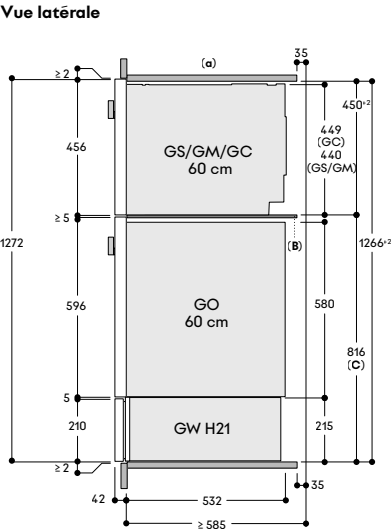
Vue latérale
