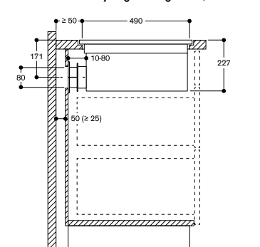
Vue de côté en recyclage sans gaines (avec CA 082 011) - installation à fleur de plan
