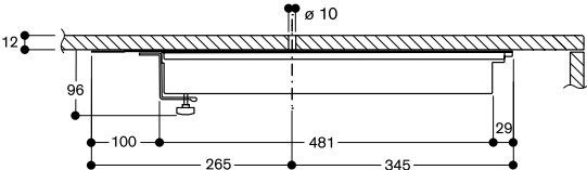
Coupe longitudinale
