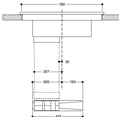
Vue de face pour CV 282 avec module de recyclage pour un système avec gaines et diffuseur d'air - installation classique
