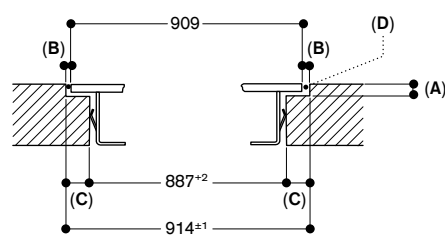
Coupe longitudinale
