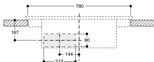
Vue de face - découpe du meuble pour recyclage installation classique
