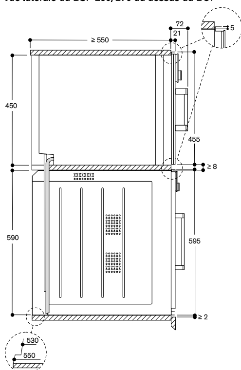
Vue latérale du BSP 260/270 au-dessus du BOP
