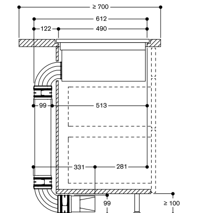
Vue de côté avec kit de recyclage pour un système avec gaines (coudes, gaines et diffuseur fournis) Profondeur plan de travail 700 mm (CA 082 071) - installation à fleur de plan
