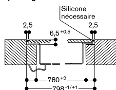
Coupe longitudinale
