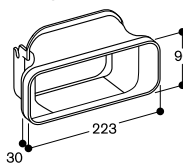
AD 851 041 : Pièce de connexion pour VL 200 pour extension avec gaine plate Ø 150 mm pour plan de travail très profond
