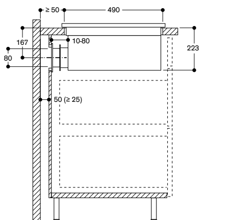
Vue de côté CV 282 111 en recyclage sans gaines
