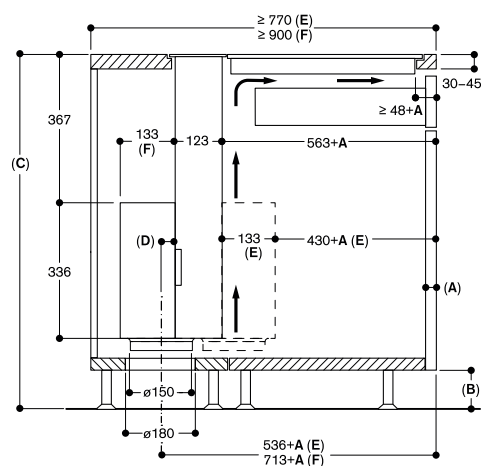
Vue latérale
