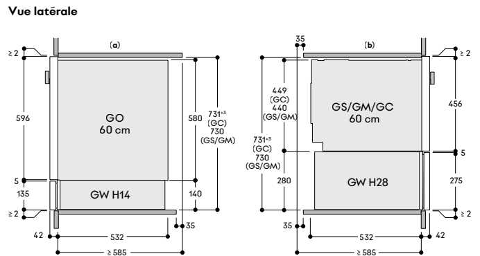
Vue latérale
