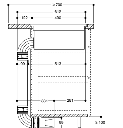
Vue de côté avec kit de recyclage pour un système avec gaines (coudes, gaines et diffuseur fournis) Profondeur plan de travail 700 mm - installation à fleur de plan
