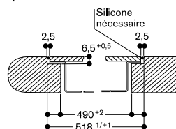
Coupe transversale
