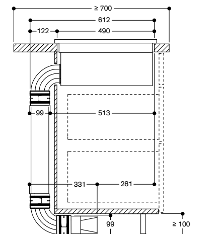
Vue de côté avec kit de recyclage pour un système avec gaines (coudes, gaines et diffuseur fournis) Profondeur plan de travail 700 mm - installation classique
