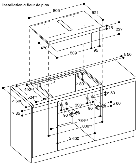
Installation à fleur de plan
