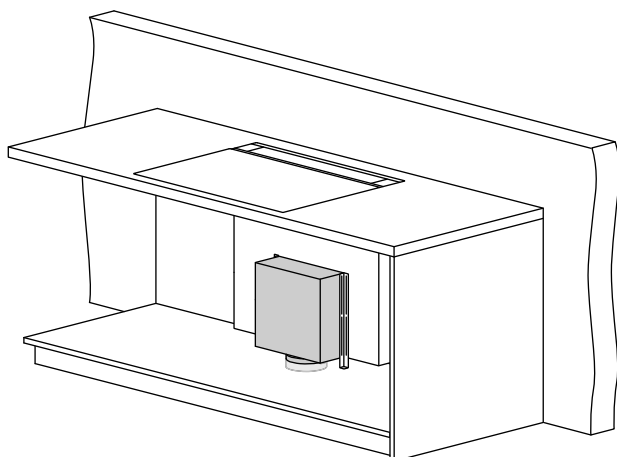
Exemple de configuration - Moteur placé à l'avant
