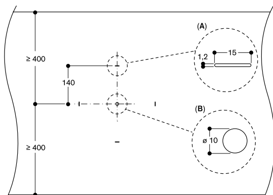
Vue de dessus - perçage du trou et marquage de la zone de cuisson
