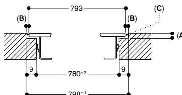
Coupe longitudinale
