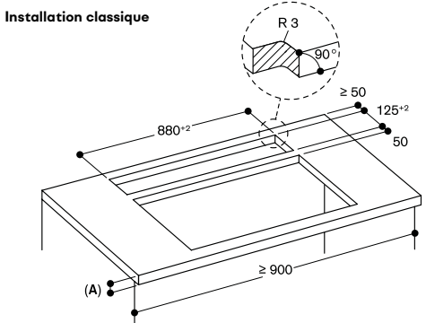
AL 200 en combinaison avec la table de cuisson sans cadre dans 2 découpes séparées Installation classique
