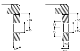
Montage des boutons de commande
