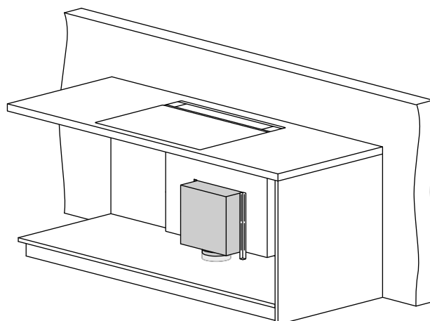
Exemple de configuration - Moteur placé à l'avant
