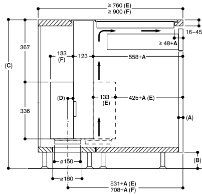
Vue latérale
