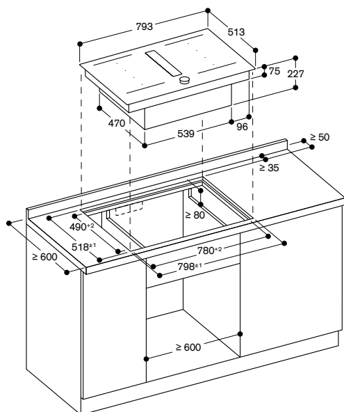
Installation à fleur de plan
