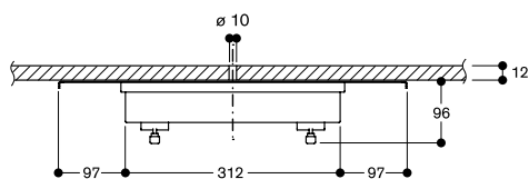
Coupe transversale
