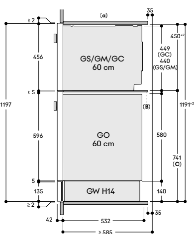
Vue latérale
