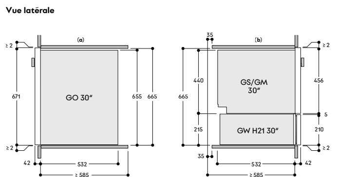
Vue latérale
