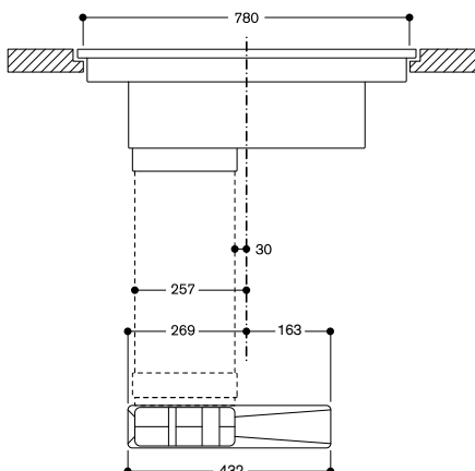
Vue de face pour CV 282 avec module de recyclage pour un système avec gaines et diffuseur d'air
