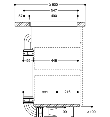
Vue de côté avec kit de recyclage pour un système avec gaines (coudes, gaines et diffuseur fournis) Profondeur plan de travail 600 mm - installation classique
