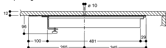
Coupe longitudinale
