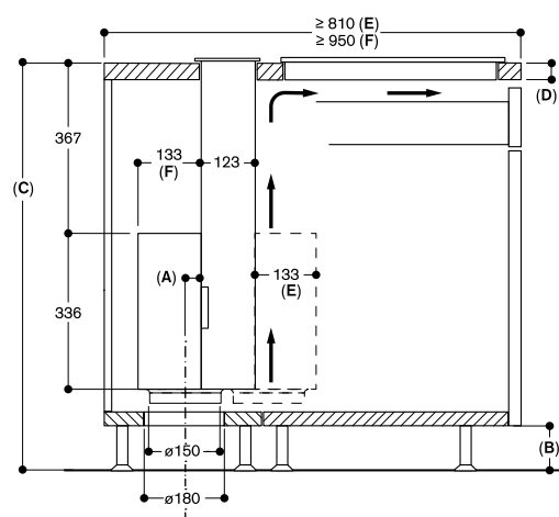
Vue latérale
