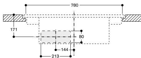
Vue de face - découpe du meuble pour recyclage à fleur de plan
